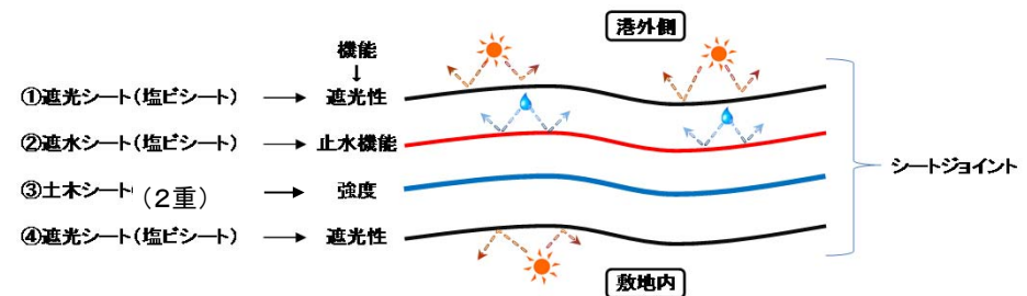
シートジョイント模式図
