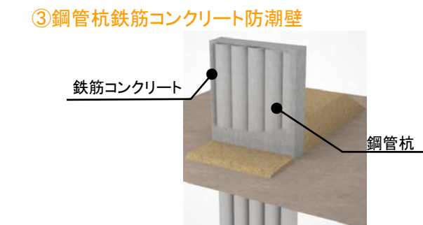
防潮堤の構造イメージ
