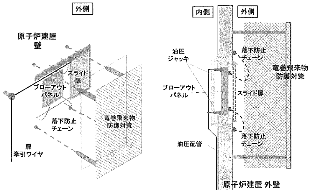
図１８．１ ブローアウトパネル閉止装置構造概略図
