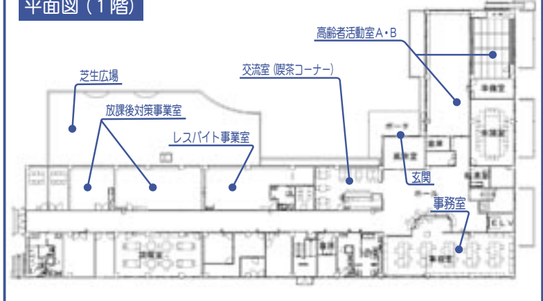
平面図(1階)
