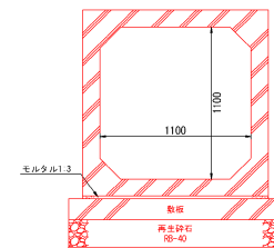
ボックスカルバート 1,100 x 1,100
