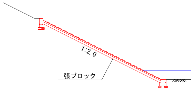
断面図 A - A
