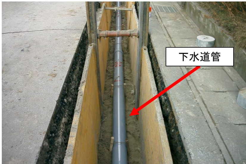
写真：開削工法
